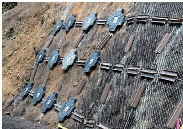
組合せ施工
