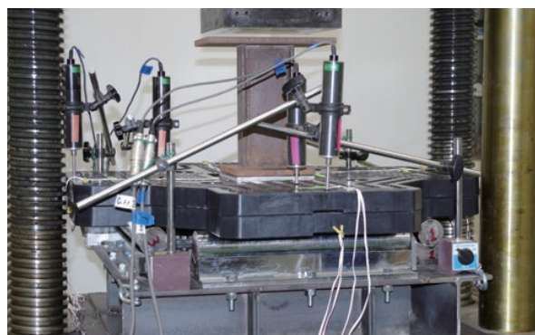
四辺支承載荷試験により適合荷重を確認
